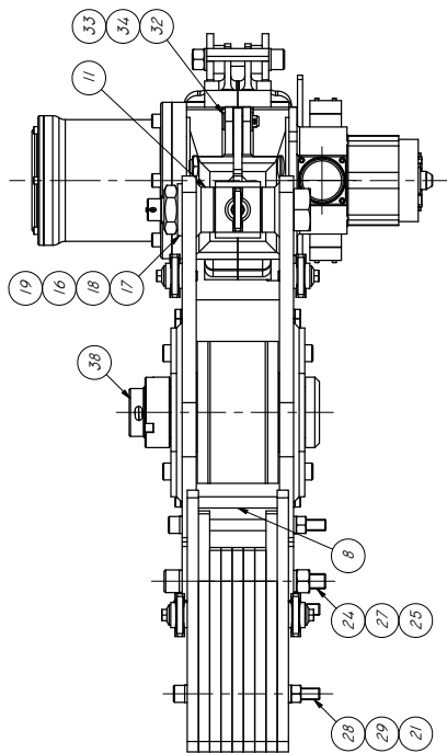
B-B ( 1:10 )
