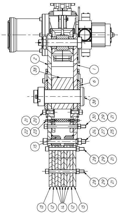
B-B ( 1:10 )
